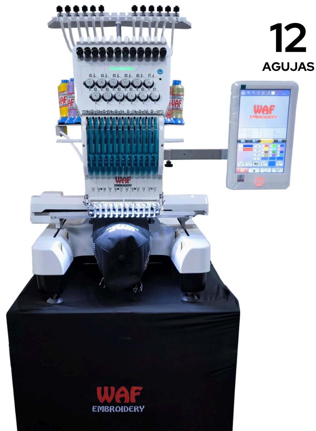
MÁQUINA DE BORDAR INDUSTRIAL WAF DE 1 CABEZA Y DE 12 CAMBIOS DE AGUJAS
